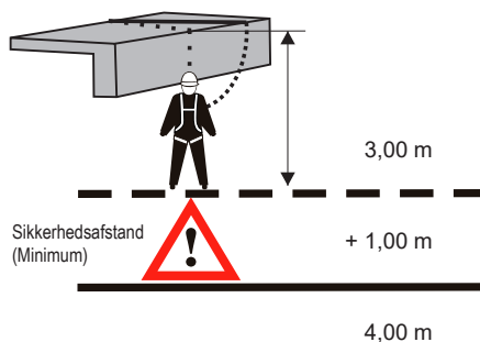
15 sidelæns fald over kanter
