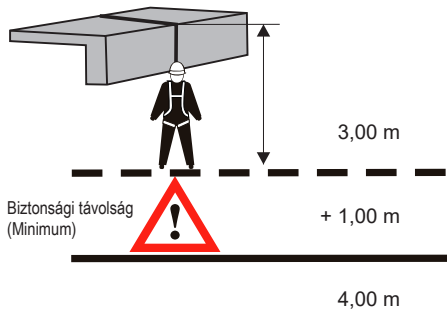
14 Merőleges irányú zuhanás peremen keresztül
