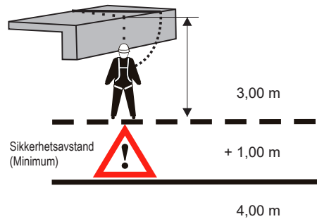
15 Sideveis fall over kant
