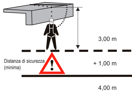
15 Caduta laterale oltre i bordi
