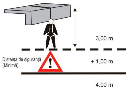
14 Cădere în unghi drept peste muchii
